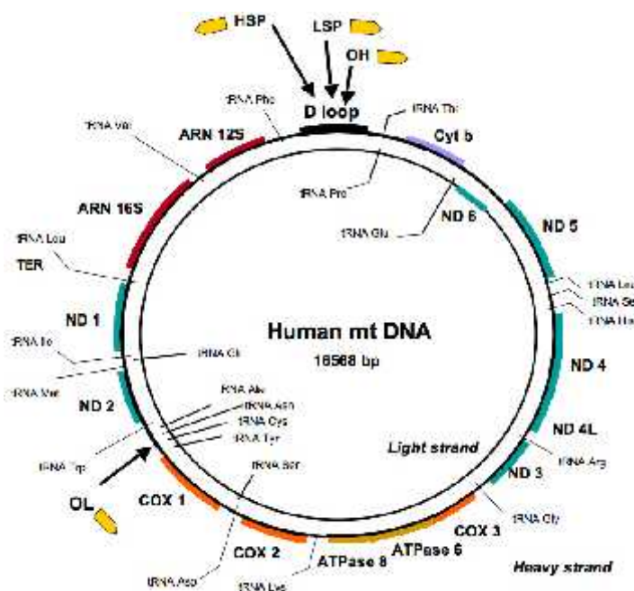
Slika 1. Ljudska mtDNA
