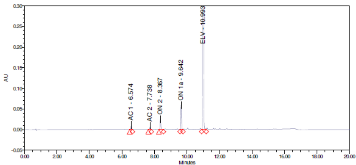
Slika D1. Kromatogram otopine IMP 1.1 pri uvjetima t = 15 \text{ min} , T = 30 \text{ }^\circ\text{C} i \text{pH} = 2,1
