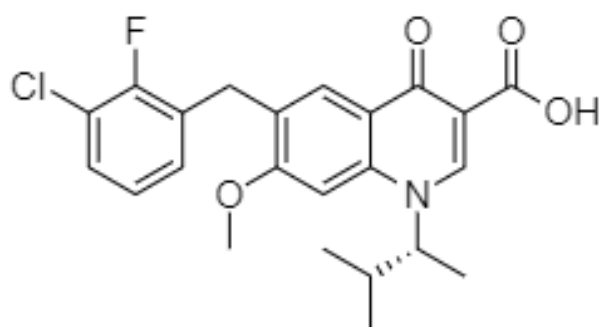
Slika 1. Struktura Elvitegravira
