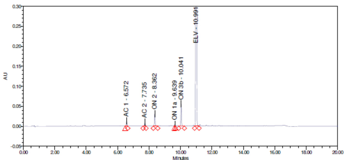
Slika D2. Kromatogram otopine IMP 1.2 pri uvjetima t = 15 \text{ min} , T = 30 \text{ }^\circ\text{C} i \text{pH} = 2,1
