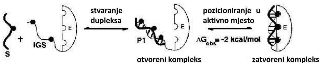
Slika 16. Upotreba vezne energije za pozicioniranje supstrata i destabilizaciju osnovnog stanja. S je supstrat koji, vežući se za IGS introna, formira P1 uzvojniju koja stvara tercijske interakcije s drugim dijelovima ribozima. Zbroj tercijskih interakcija bi bio -11,0 \text{ kcal mol}^{-1} , ali je uočena tercijska stabilizacija samo 2 \text{ kcal mol}^{-1} .
