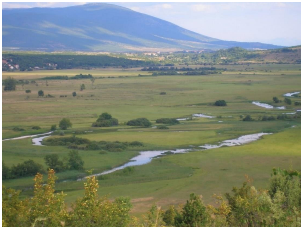
Sl. 18. Močvarna zona 1a i pogled na Cetinsko-Paško polje
