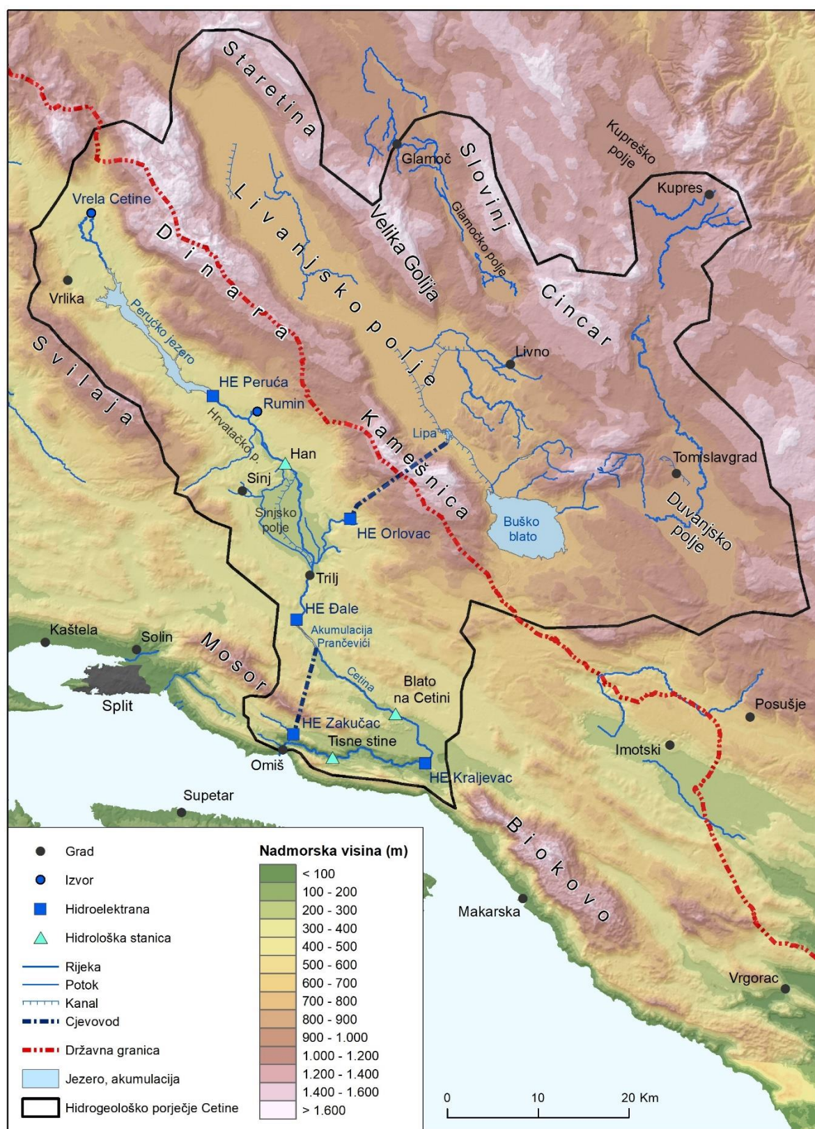
Sl. 1. Hidrogeološko porječje Cetine određeno prema Provedbenom planu obrane od poplava (2014)
