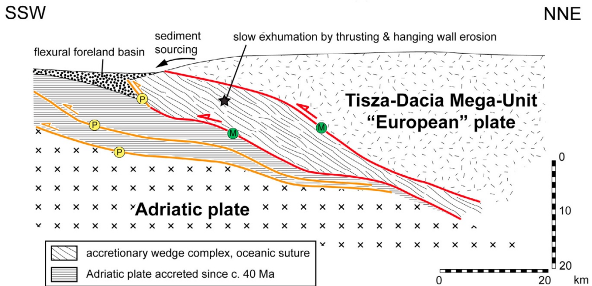
Slika 6.5: Shematski prikaz geotektonske situacije duž kontakta Adrije i Tisijske od kasnog paleocena do ranog oligocena (59–30 Ma); s položajem Sava zone (oceanic suture) , rubnog predgorskog bazena ( flexural foreland basin ), te smjera donosa detritusa u bazen ( sediment sourcing ). M – mastrichtijska sutura (70–65 Ma); P – srednjoeocenske do donjooligocenske navlake ( thrusts/"nappe" ) (40–30 Ma). Preuzeto iz USTASZEWSKI et al. (2010).
