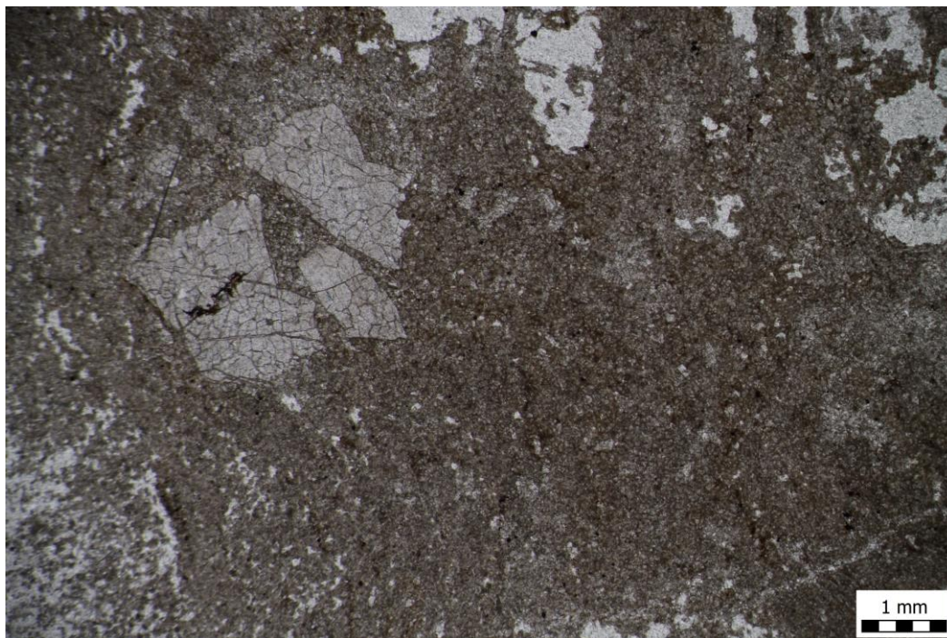
Slika 10. Mudstone do wackestone mikrofacijes s rekristaliziranim fragmentima druge/starije stijene (uzorak B4b, zona 2)
