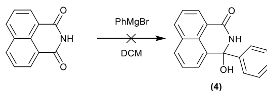
Slika 30. Pokušaj provođenja Grignardove reakcije naftalimida i fenilmagnezijevog bromida.
