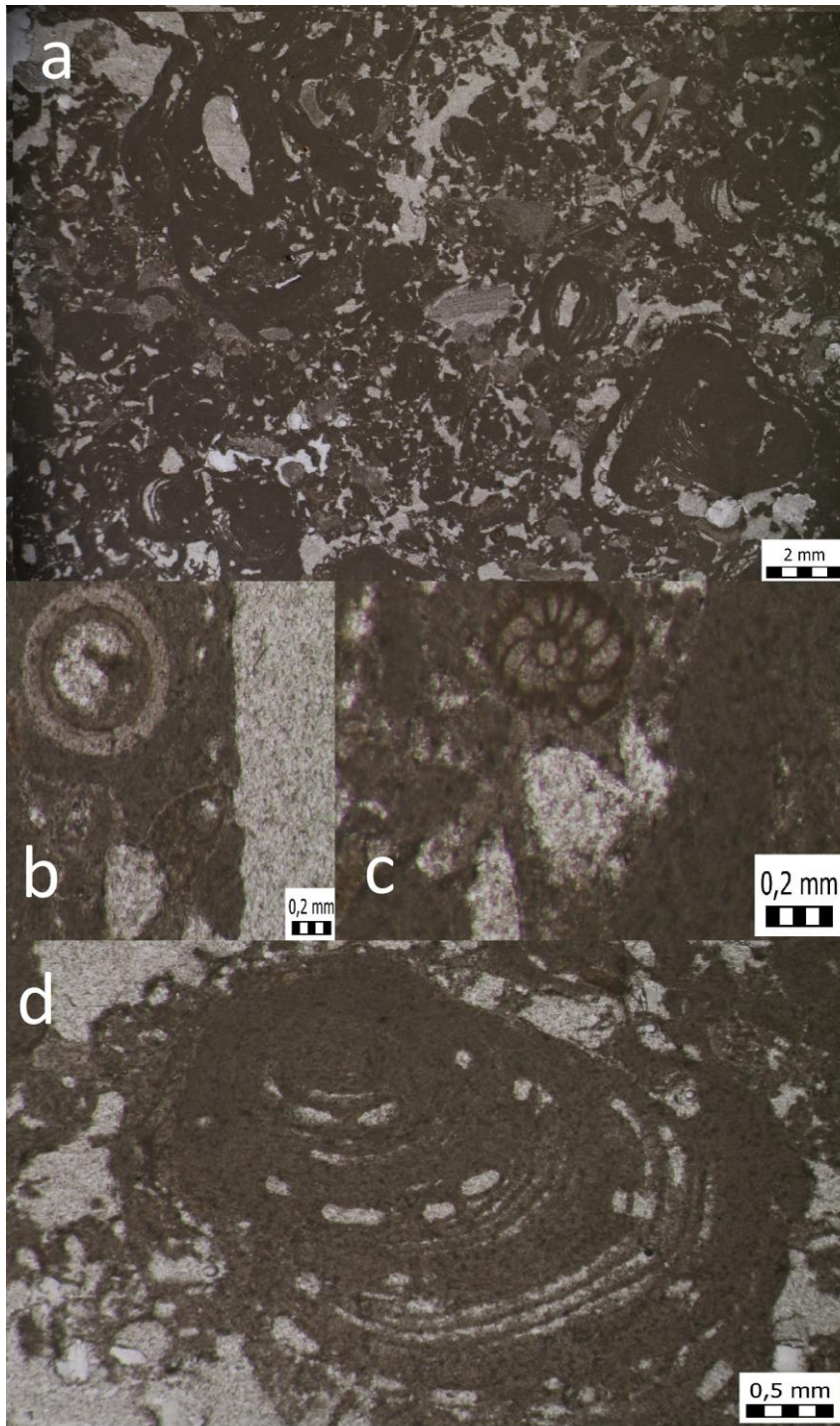
Slika 18. Mikrofotografija u prolaznom svijetlu preparata na lokalitetu šumskog puta prema Veternici; a) kalkarenit s crvenim algama b) poprečni presjek skafoпода c) ekvatorijalni presjek foraminifere d) rodolit s konceptakulima, rod Lithothamnion
