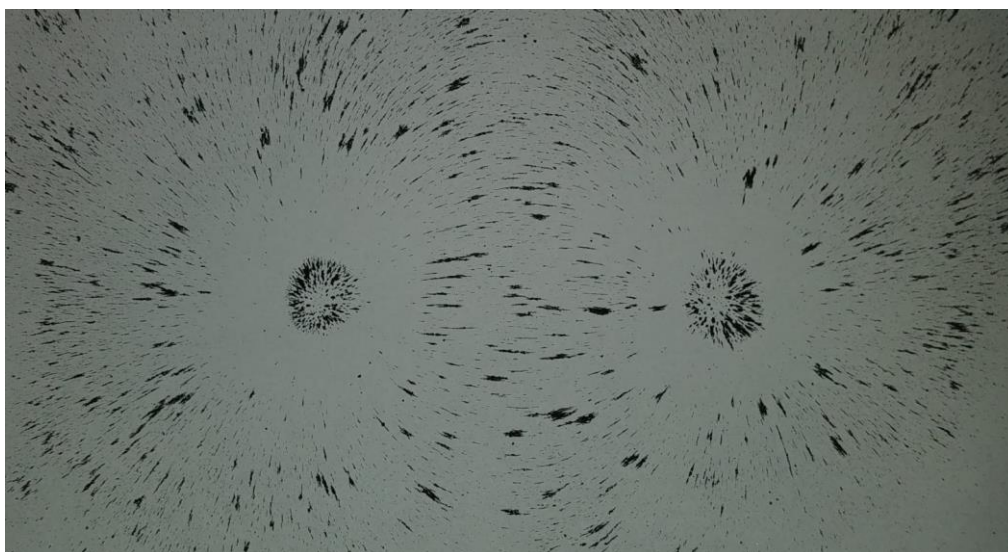
Slika 24 Silnice magnetskog polja magneta na papiru
