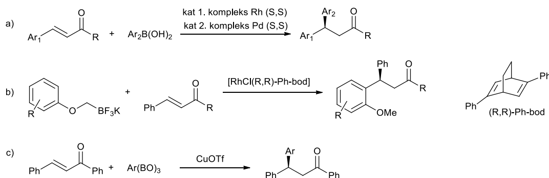
Slika 31. Shematski prikaz reakcija pripreme \beta,\beta -diaril-ketona katalizirane kompleksima prijelaznih metala
