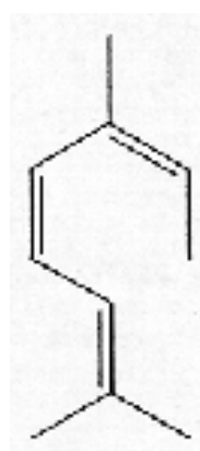
aloocimen
