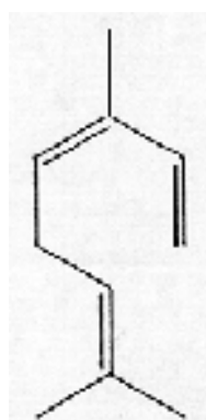
\beta -ocimen
