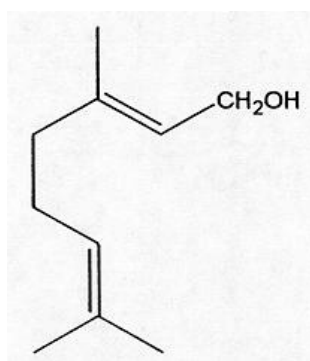
geraniol
