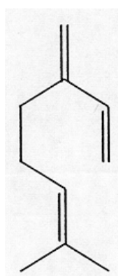
mircen
