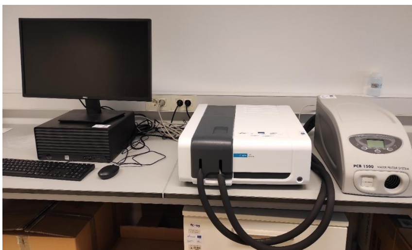
Slika 23. Cary 60 UV-Vis spektrofotometar
