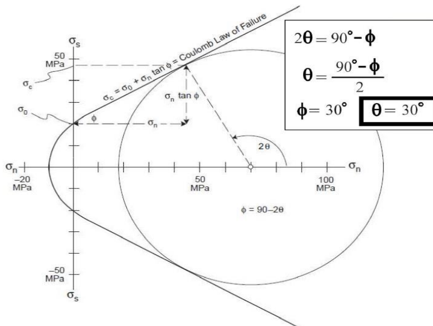
Slika 3–6. Mohrova kružnica posmičnog naprezanja nadopunjena sa anvelopom sloma za tipični pješčenjak (DAVIS & REYNOLDS, 1996; TOMLJENVIĆ, 2015)
