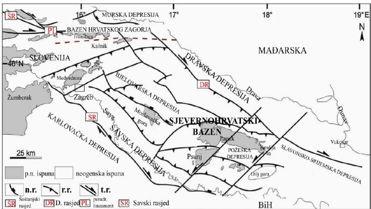
Slika 3-3. Strukturna karta rasjeda i karta prikaza podloge paleogena i neogenske ispune na području hrvatskog dijela panonskog bazena ( Pavelić i Kovačić, 2018 prema Márton, 2002 i Ustaszewski, 2004)
