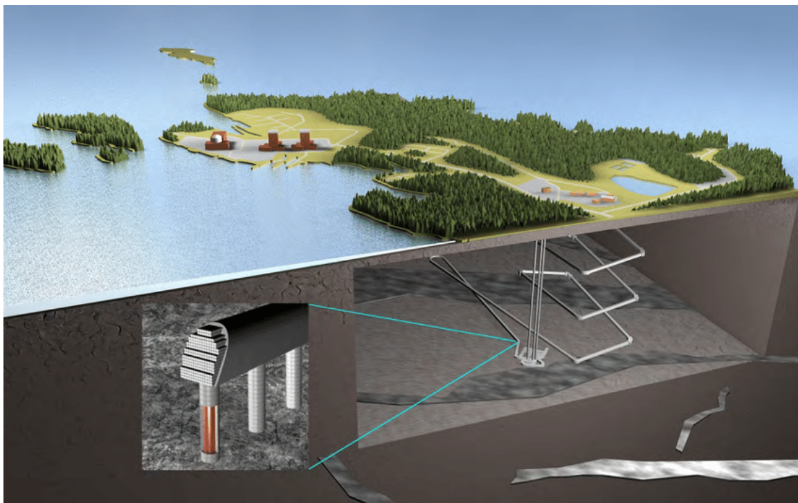
Slika 4-1 Švedski model odlaganja VRAO (McEwen i dr., 2012)
