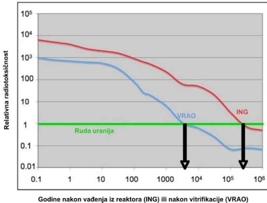
Slika 3-1 Pad radiotoksičnosti kao rezultat radioaktivnog raspada prikazan kao funkcija vremena za ING i VRAO (Uroić, 2019).
