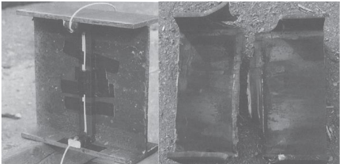
Slika 6-30 C-4 eksploziv pričvršćen na čeličnu gredu (slika lijevo) i prikaz štete koju je eksploziv napravio (slika desno) (Weickert, 1998)
