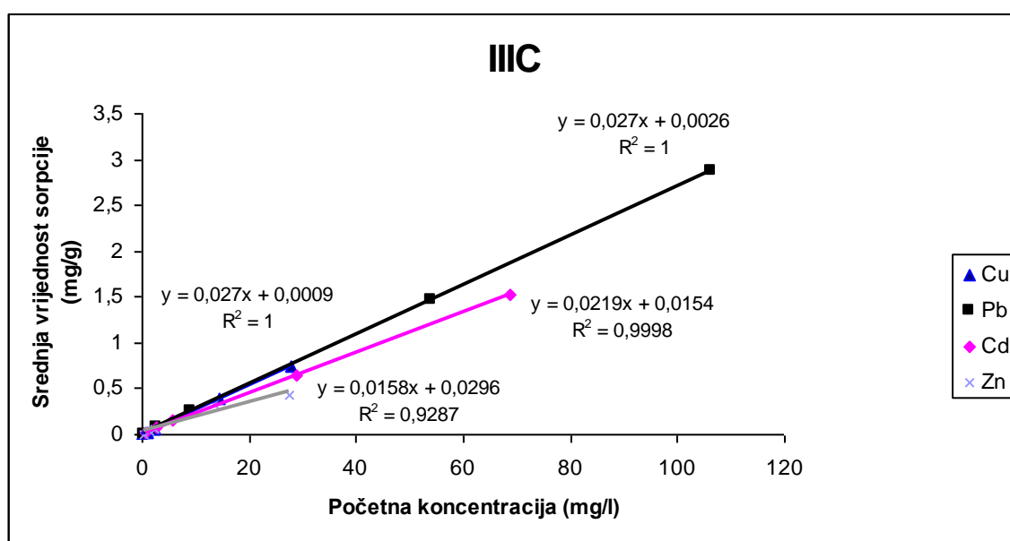
Slika 16. Graf izoterme za Pb, Cu, Cd i Zn za horizont IIIC
