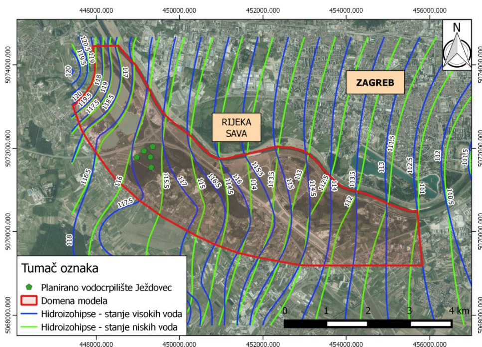
Slika 5.3 Domena modela
