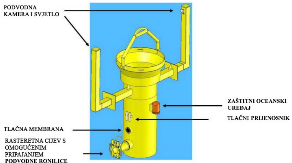
Slika 6-4. Sastavni dijelovi usisnog modula (Stave et al., 2014).
