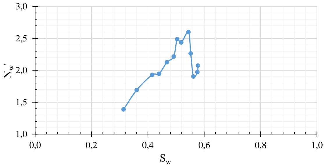
Slika 4-8. Grafičko eliminiranje odskočnika kod određivanja Coreyevog eksponenta N_w .
