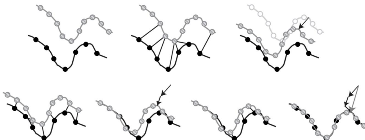
Slika 3.3. ICP algoritam
