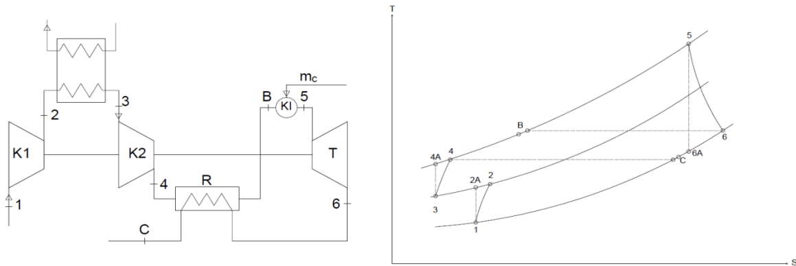
Slika 29. Shema i T-s dijagram otvorenog sustava plinske turbine u kombinaciji sa međuhlađenjem i regeneratom toplinu
