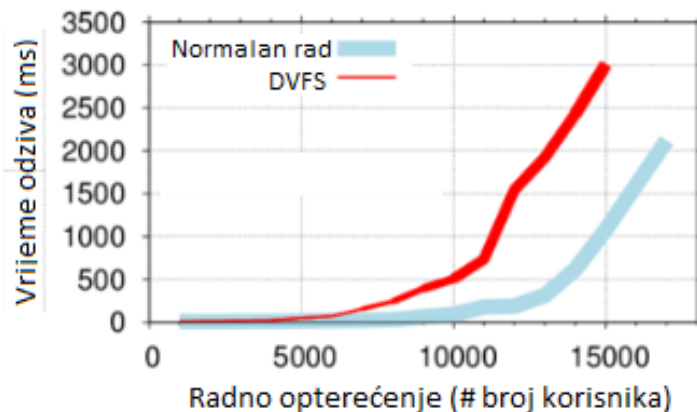
Slika 4.3 Vrijeme odziva sustava se povećava s uključenim DVFS-om[34]
