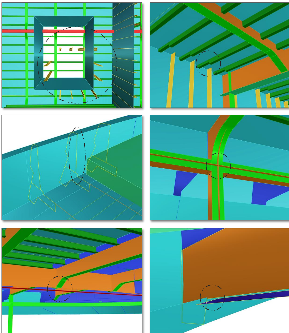
Slika 4.9. Greške geometrijskog modela – Neusklađenost [4].
