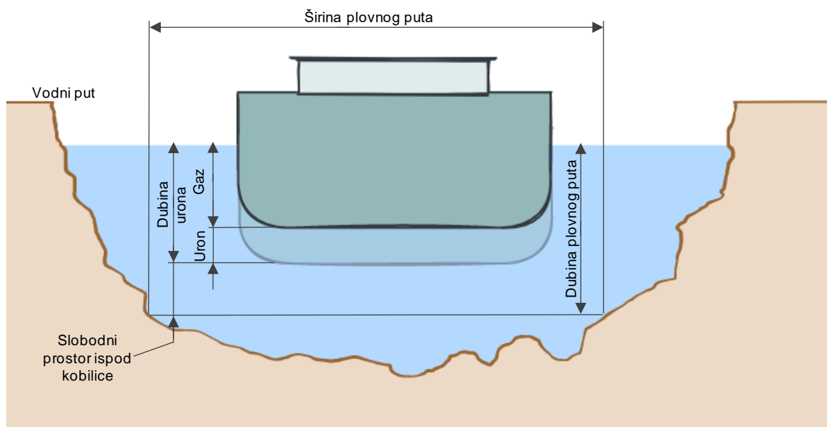
Slika 2.1. Odnos dimenzija plovnog puta [2].
