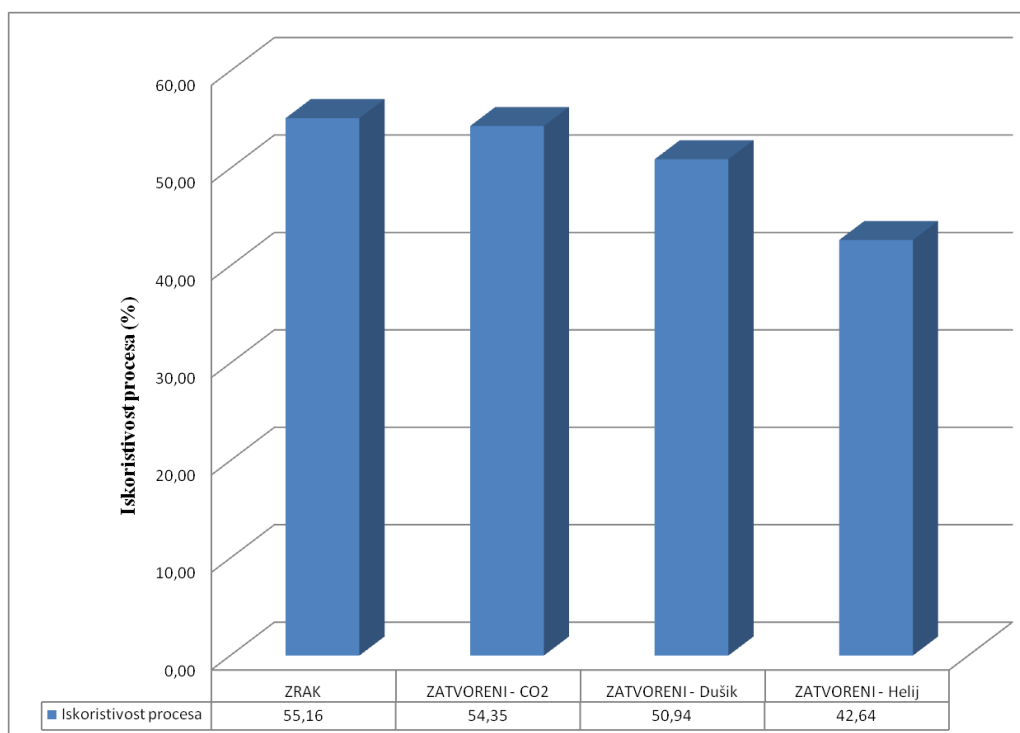
Slika 15. Grafički prikaz i usporedba iskoristivosti sustava sa regeneratorom topline
