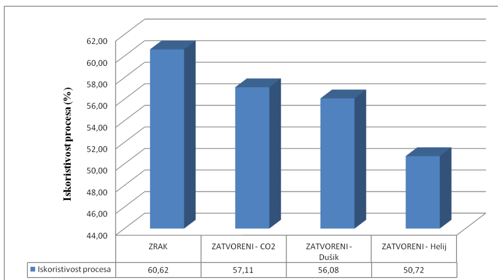
Slika 38. Grafički prikaz i usporedba iskoristivosti kombinacije sustava sa međuhlađenjem i regeneratorom topline
