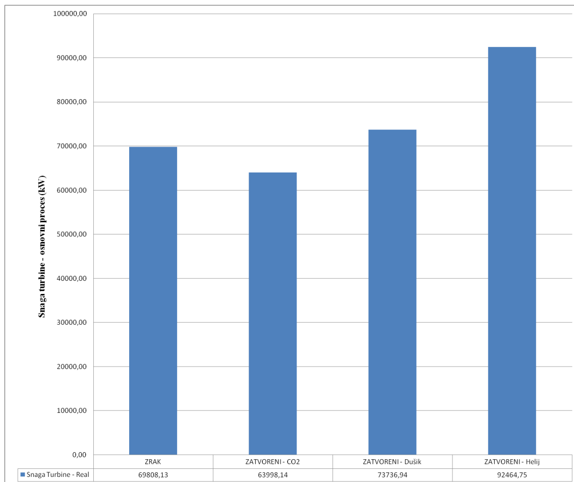
Slika 53. Grafički prikaz snage turbina u osnovnom sustavu bez nadogradnji
