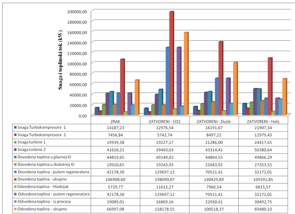
Slika 46. Grafički prikaz i usporedba vrijednosti kombinacije sustava sa naknadnim izgaranjem, regeneratorskom i međuhlađenjem
