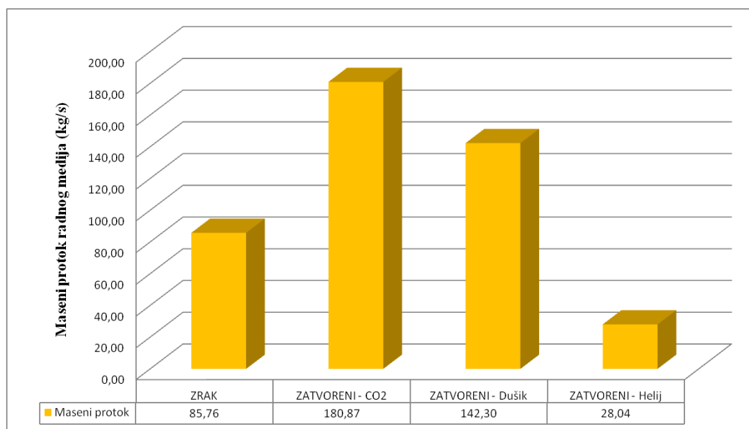
Slika 20. Grafički prikaz i usporedba vrijednosti masenih protoka sustava sa međuhladnjakom
