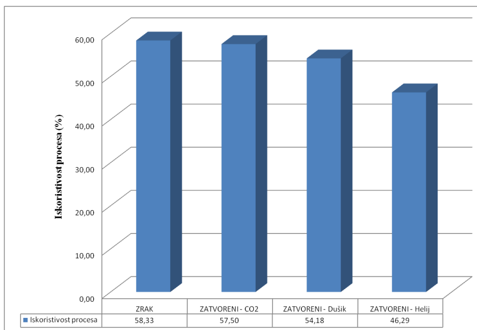
Slika 33. Grafički prikaz i usporedba iskoristivosti kombinacije sustava sa međuhlađenjem i regeneratorom topline
