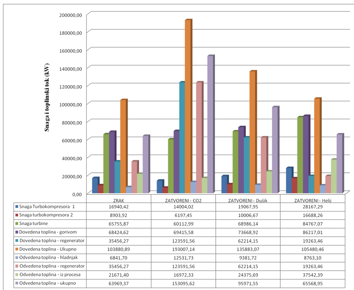
Slika 31. Grafički prikaz i usporedba vrijednosti kombinacije sustava sa međuhlađenjem i regeneratorom topline
