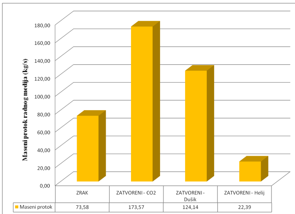
Slika 27. Grafički prikaz i usporedba vrijednosti masenih protoka sustava sa naknadnim izgaranjem
