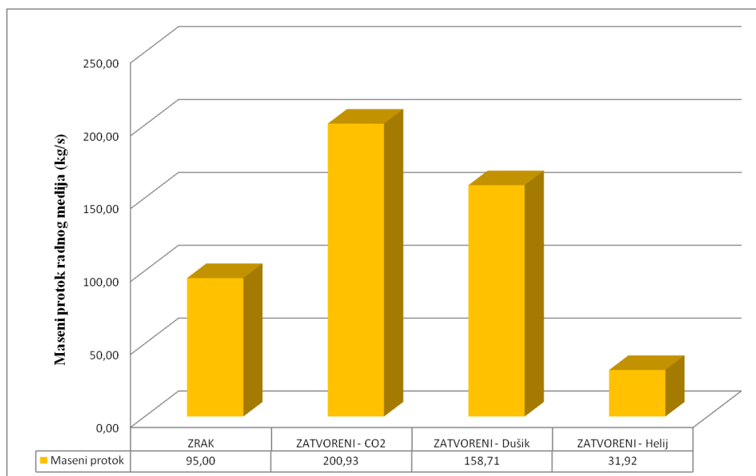
Slika 14. Grafički prikaz i usporedba vrijednosti masenih protoka sustava sa regeneratorskom toplinom
