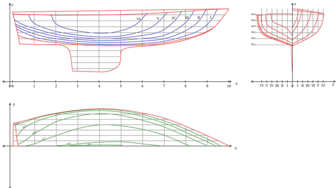
Slika 1.2 Nacrt linija jedrilice klase L5
