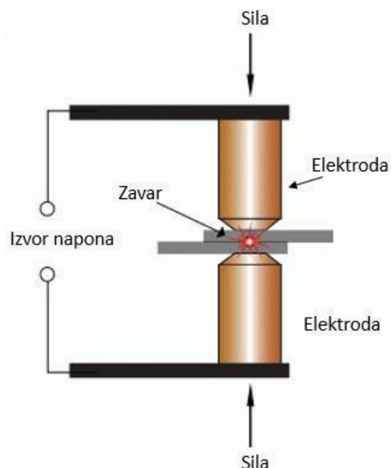
Slika 12. Prikaz direktnog točkastog zavarivanja [14]
