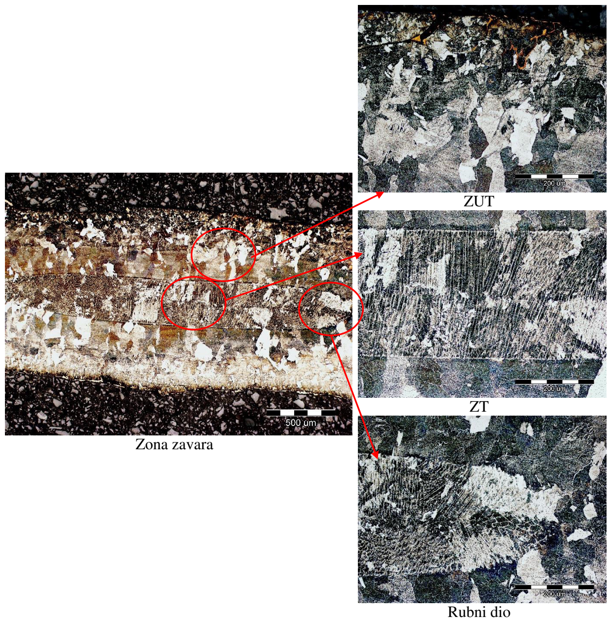
Slika 28. Zona taljenja i zona utjecaja topline u zavaru uzoraka iz trake uzimane s vozila Peugeot
