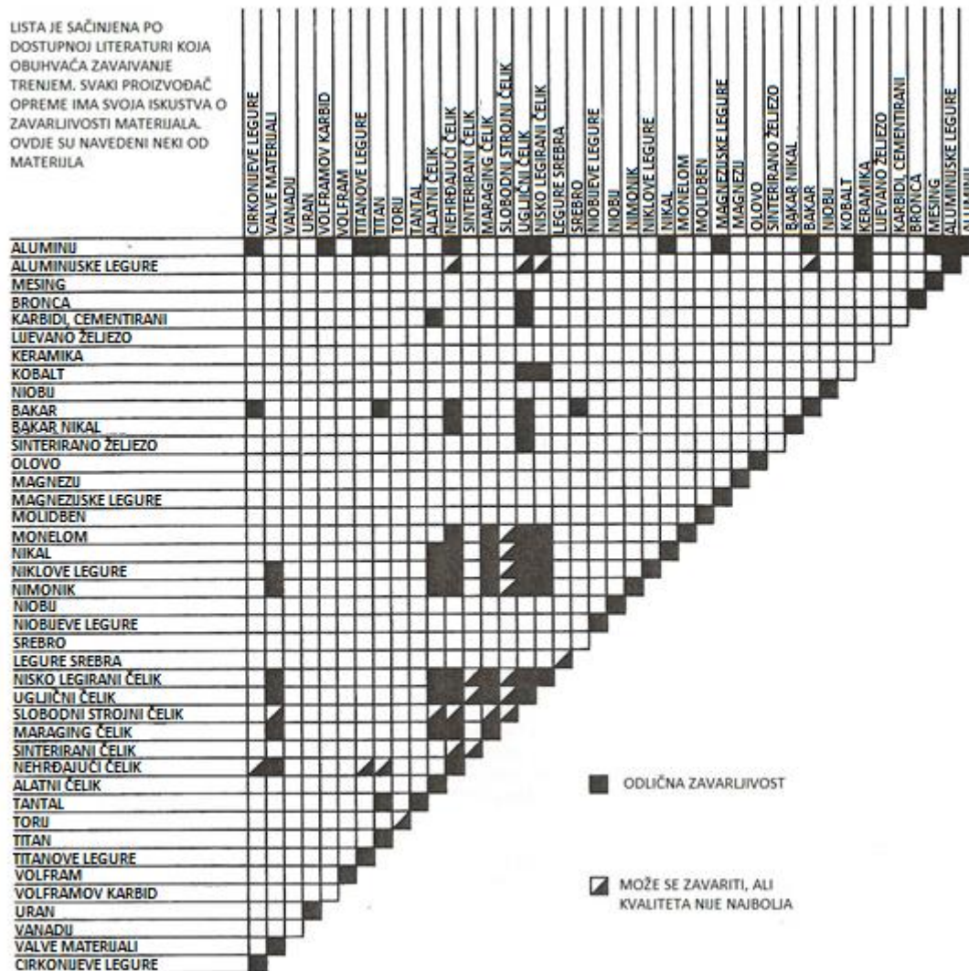
Tablica 3. Kombinacije materijala i njihova zavarljivost postupkom zavarivanja trenjem [20]
