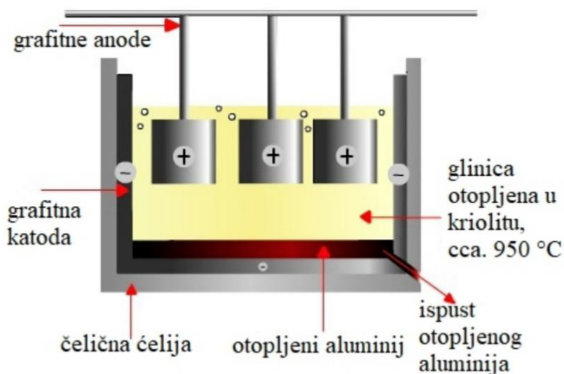
Slika 8. Hall-Héroultov proces [36]
