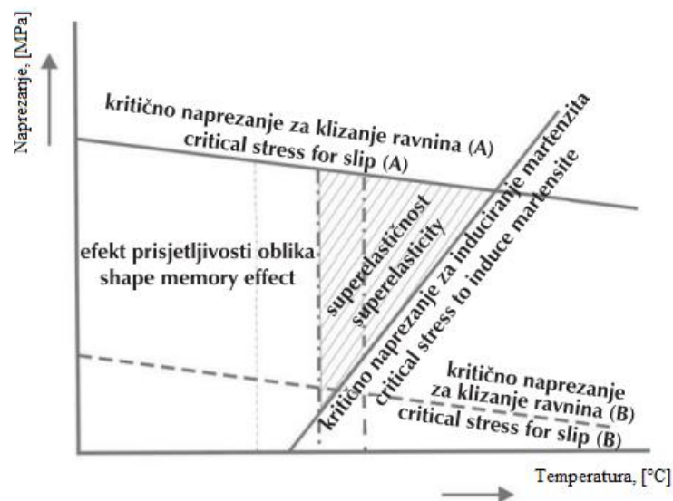
Slika 10. Shematski prikaz područja superelastičnosti i efekta prisjetljivosti oblika u ovisnosti naprežanja i temperature [6]
