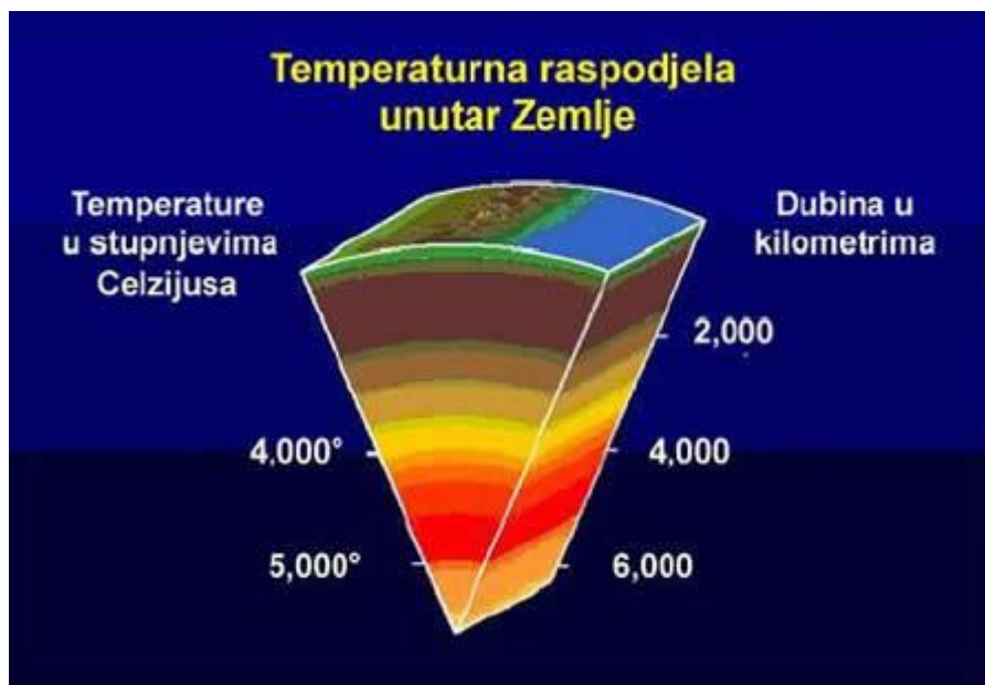
Slika 4. Presjek Zemlje s temperaturnom raspodjelom (izvor: http://www.obnovljivi.com/geotermalna-energija/67-iskoristavanje-geotermalne-energije-u-energetici?showall=1 )
