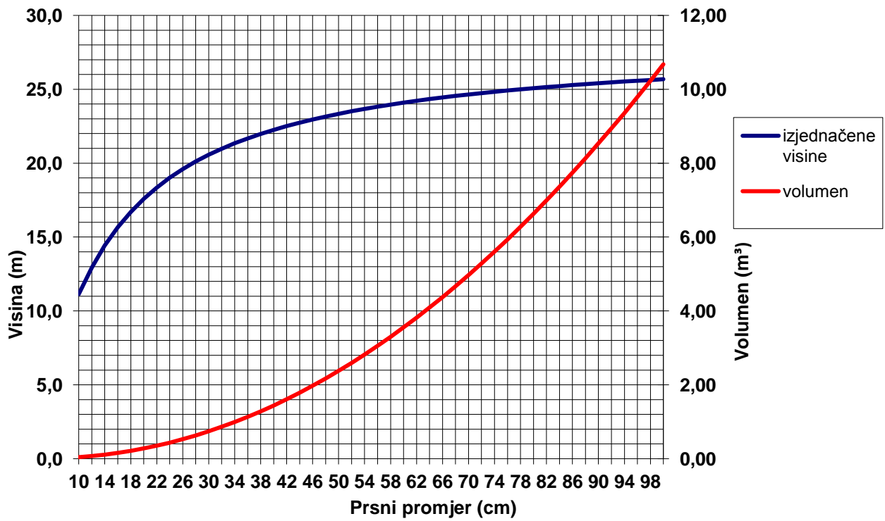
Grafikon 1. Visinska krivulja i tarifa za vrbu, ploha 1
