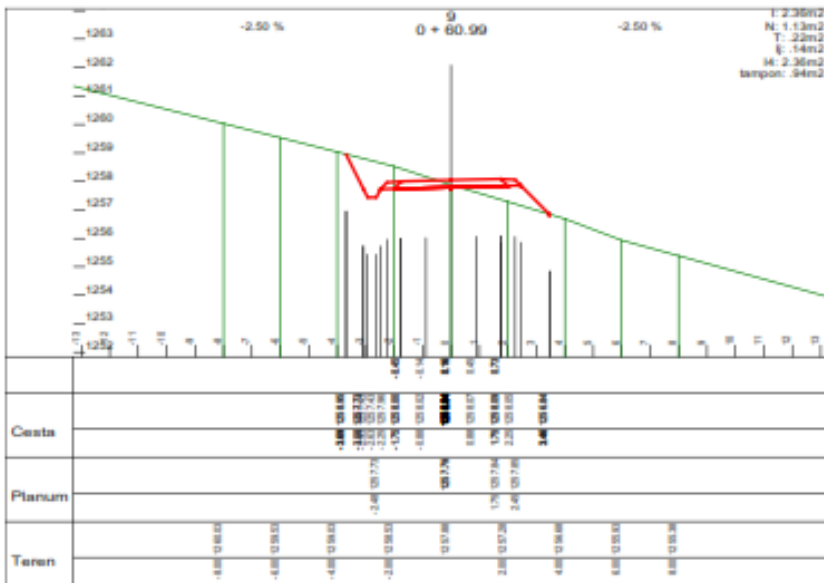
Slika 11. Grafički prikaz crtanih poprečnih profila 8 – 11 šumske ceste „Maričića vrh“
