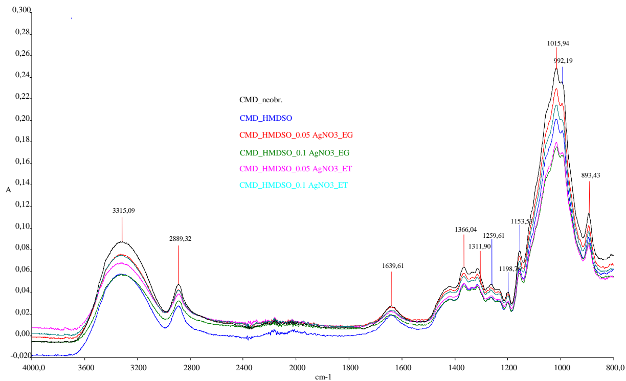
Slika 44. FTIR-ATR analiza funkcionalnih skupina modalnih vlakana obrađenih s HMDSO i AgNO 3
