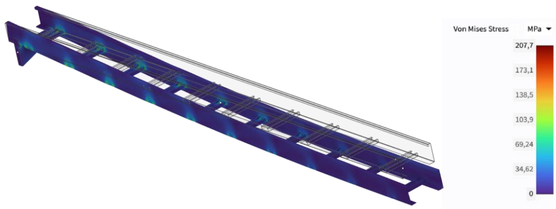
Slika 3.10 Simulacija polovice ljestava prikaz ekvivalentnog Von Misesovog naprezanja u MPa
