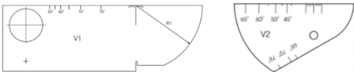
Slika 4.6 Kalibracijski blokovi V1 i V2 [8]
