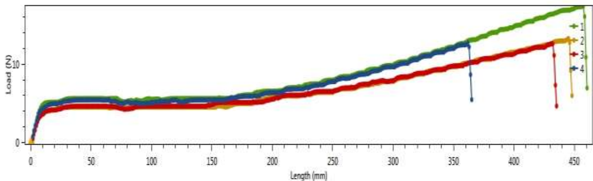
4.21 Rezultati ispitivanja na kidalici [25]
