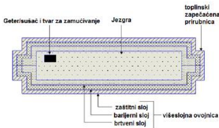
Slika 4.5.3.2 Detalj VIP-a [24]
