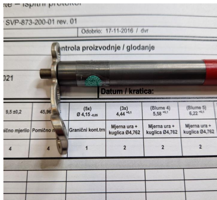
Slika 39. Provjera sa graničnim kontrolnim zaticom
