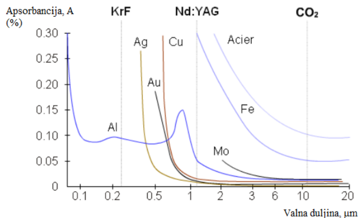
Slika 3.7 Apsorpcijski koeficijent pojedinih metala [18]
