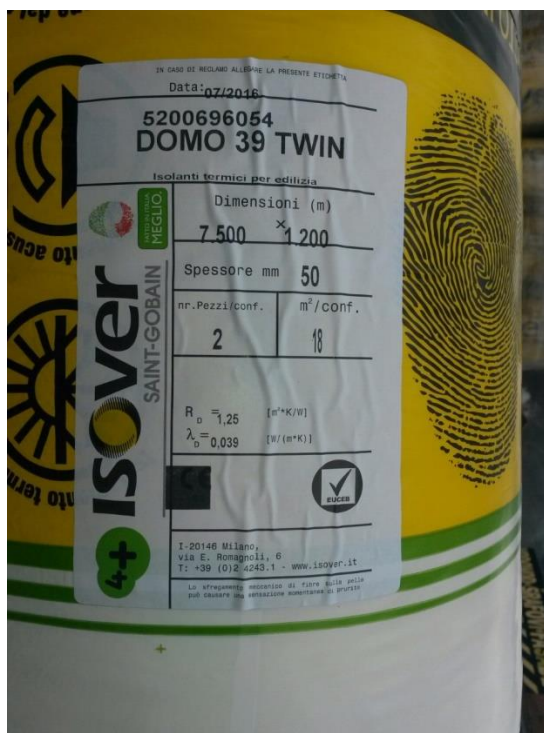
Slika 3.2.1. Prikaz koeficijenta toplinske provodljivosti \lambda = 0,039 (W/mK) na deklaraciji mineralne staklene vune proizvođača Isovover – Saint Gobain
