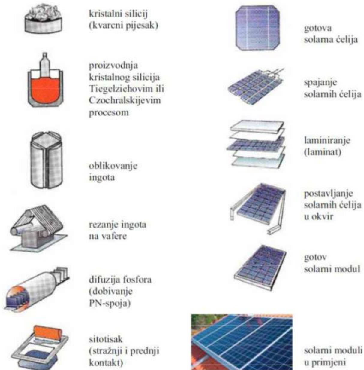
SLIKA 3.3. Postupak proizvodnje solarnih ćelija i FN modula [4]
