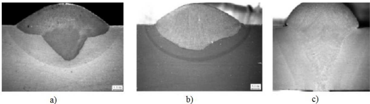
Slika 10.6 Utjecaj razmaka žice na zavar: a) i b) isto podešeni parametrima zavarivanja, ali različiti razmaci žice, c) optimalno podešeni parametrima za maksimalno uvarivanje [30]
