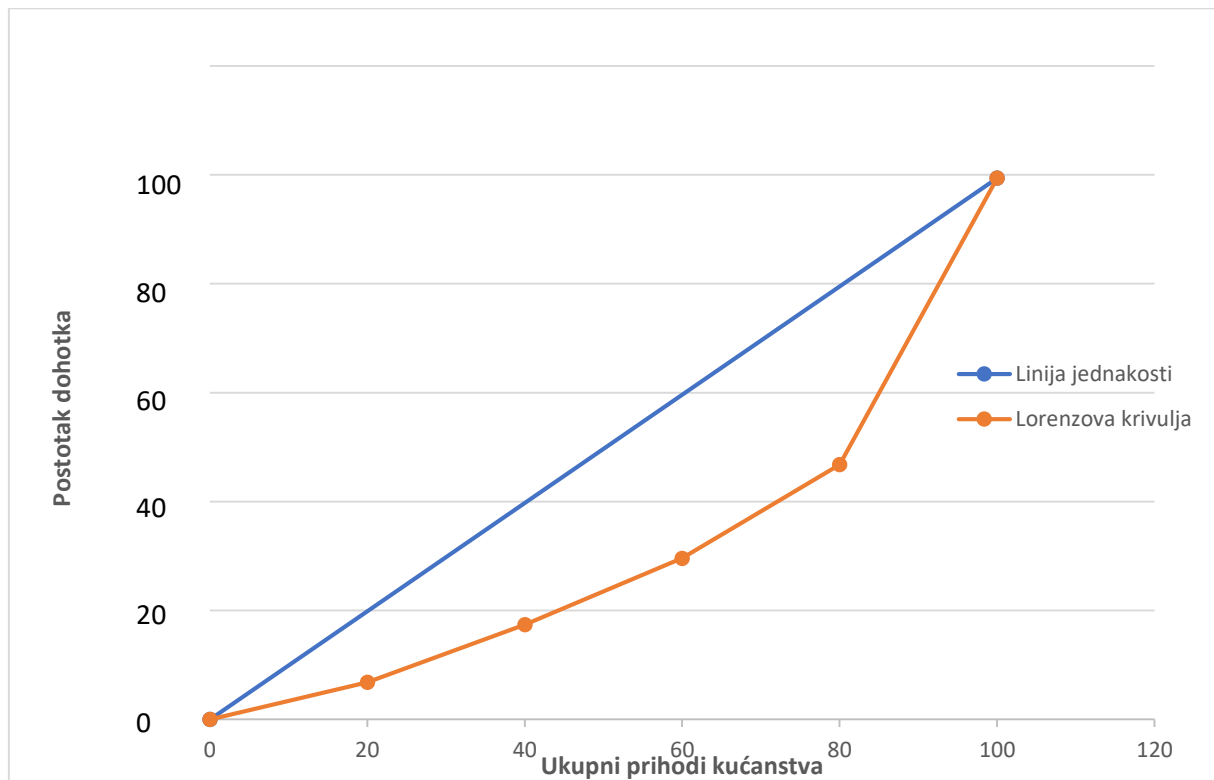
Slika 1. Lorenzova krivulja
