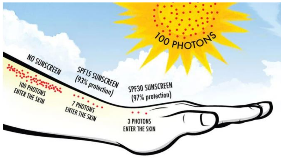
Slika 2 Prolaz fotona
