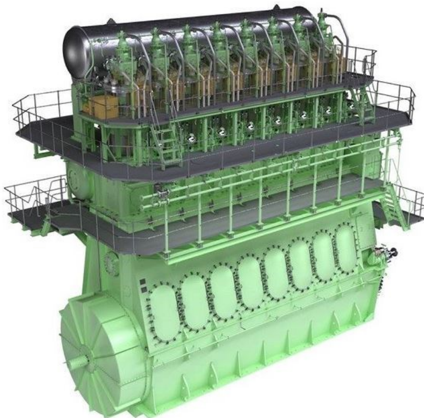
Slika 2. Sporookretni dvotaktni motor s križnom glavom
