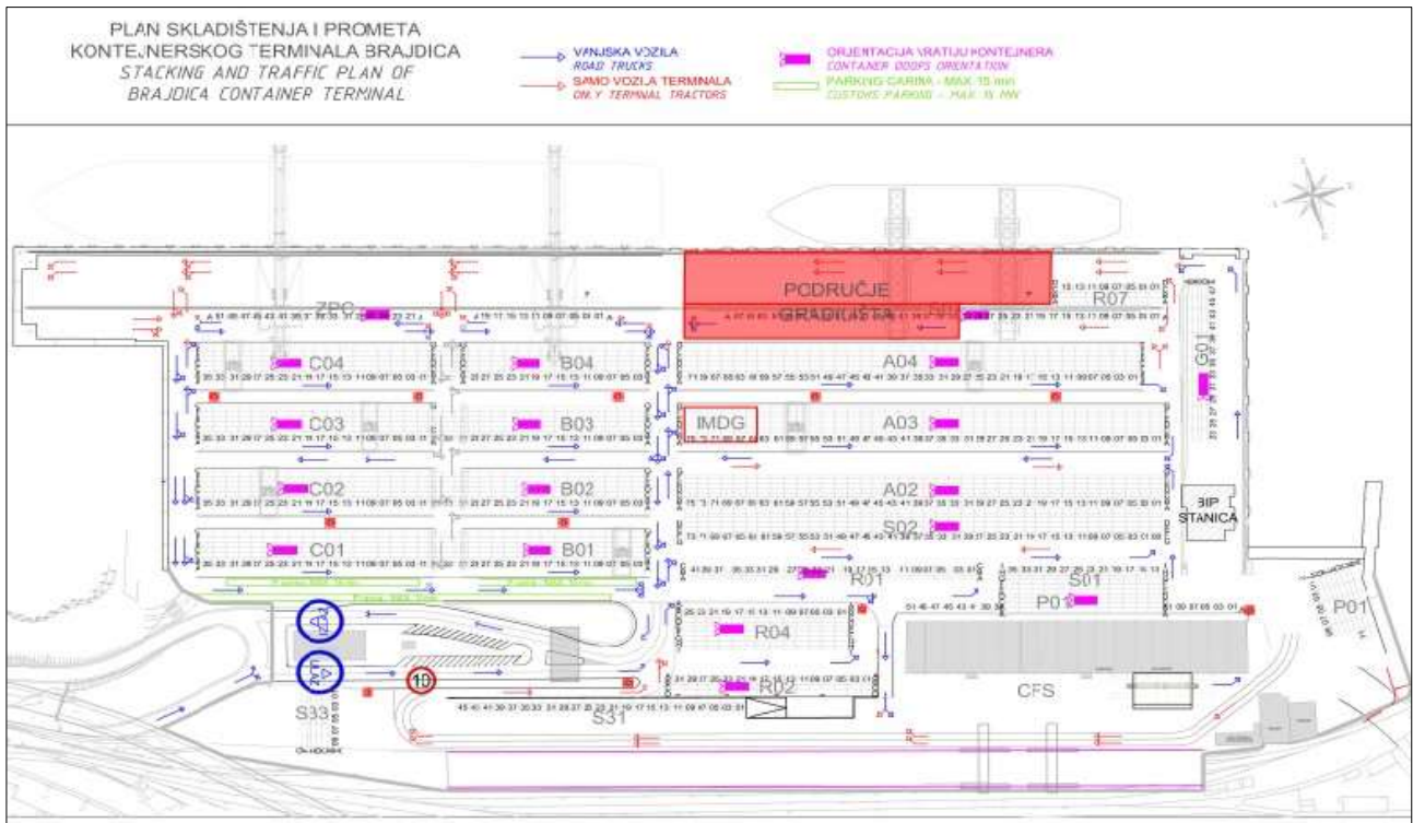
Slika 12 - Slika Plan skladištenja i prometa AGCT Brajdica
