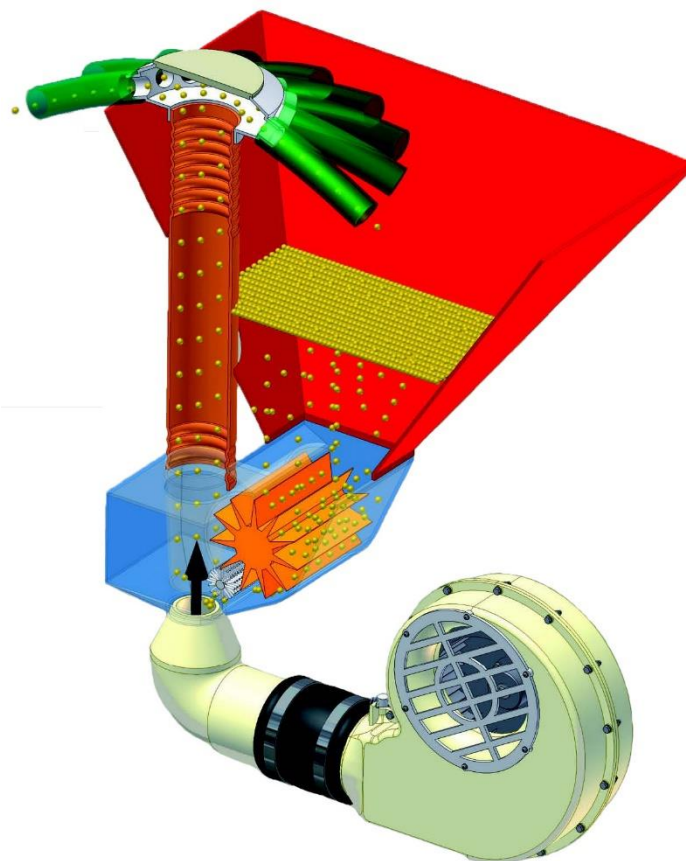
Slika 7. Shematski prikaz rada sijačice VogelNoot Power Drill A300 (Izvor: V. Miloš)
