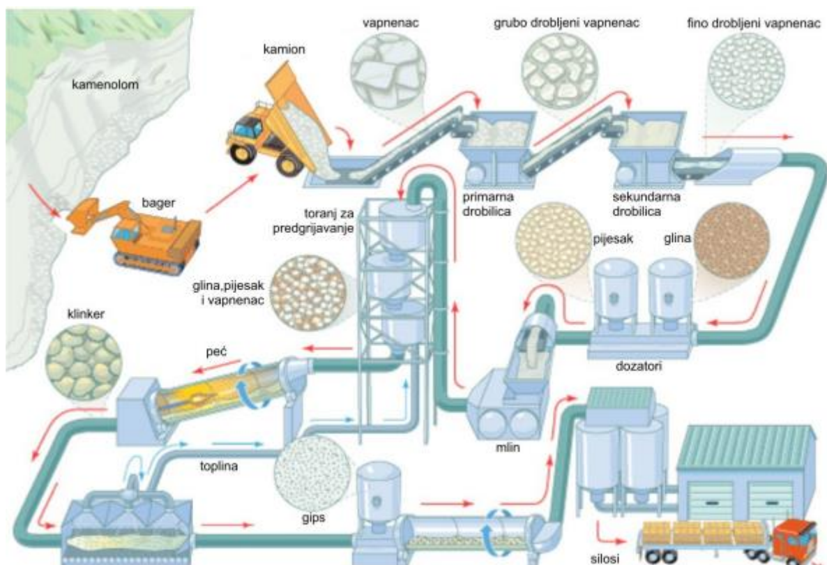
SI. 3 Suvereni način proizvodnje cementa [2]
