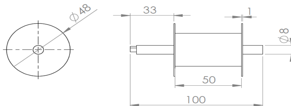
SLIKA 30. Nacrt i bokocrt bubnja s osnovnim dimenzijama
