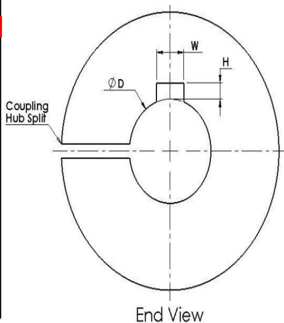
SLIKA 37. Dimenzije klinova [17]
